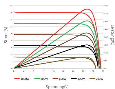
Strom-Spannungs- und Leistungs-Spannungs-Diagramme (445W)
